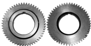
D235 - ENGRENAGEM EIXO VIRABREQUIM VOLANTE 7CV
