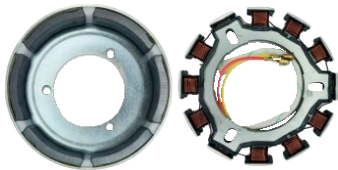
D166 - ALTERNADOR COMPLETO 5/7/10/13CV
